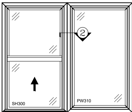
DH300 & PW310
